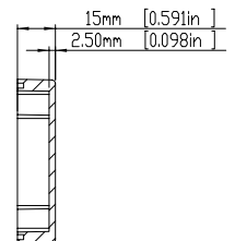
SECTION B-B SCALE 2 : 3
