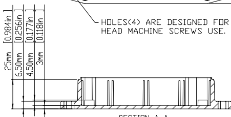
SECTION A-A SCALE 2 : 3
